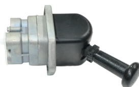
55175VLT пневмокран тормозной ручной [9617231020] M16x1.5 6.5bar MAN
