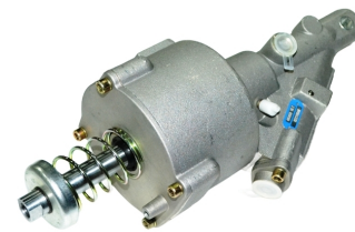
05459VLT ПГУ 100mm [622109AM] SCANIA/DAF
