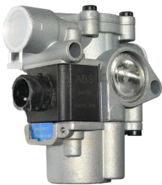
05063VLT клапан элект.магнитный ABS байонет [4721950160] 24V, воздух 2*M22x1,5 VOSS, сенсор BAJONET DIN72585
