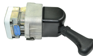
05890VLT пневмокран ручного тормоза [DPM66A] MB
