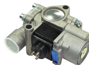
05155VLT клапан магнитный ABS [4721950150] 24V воздух 2*M22x1,5 , сенсор M27x1
