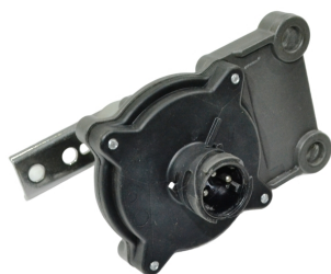
05662VLT пневмокран уровня пола [0504002114] MAN
