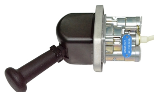
05095VLT пневмокран ручного тормоза P2max=5.9 BAR/Port threads:M16x1.5mm [9617230210] SCANIA/DAF
