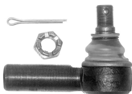
06308VLT наконечник рулевой RHT M24x1,5 / M18x1,5 L=105mm, K=22 [0023301335]
