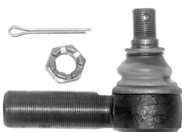
06398VLT наконечник рулевой LHT M28x1,5 / M20x1,5 L=115mm, K=26 [04688942]
