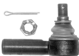
06610VLT наконечник рулевой RHT M30x1,5 / ... L=141mm, K=32 [0013309935]
