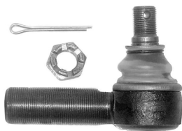
06314VLT наконечник рулевой RHT M30x1,5 / M20x1,5 L=120mm, K=26 [1142173] DAF/IVECO/MAN/MB
