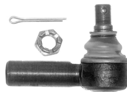
06748VLT наконечник рулевой LHT M30x1,5 / M24x1,5 [180341406010] увеличенный конус
