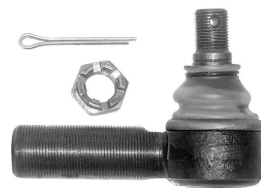
06306VLT наконечник рулевой LHT M24x1,5 / M18x1,5 L=105mm, K=22 [0003309835] [01084 VLT]
