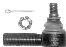
06379VLT наконечник рулевой RHT M32x1,5 / M24x1,5 L=140mm, K=30 [5001867774]
