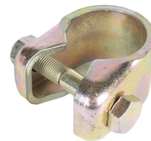
06733VLT хомут рулевой тяги 42mm (хомут+2 болта+2 гайки) КАМАЗ-6520 [6520-3414064-11] широкий на 2 болта
