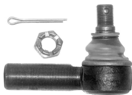
06313VLT наконечник рулевой RHT M30x1,5 / M27x1,5 L=158mm, K=32 [0004604848], MB ACTROS [17311 VLT]
