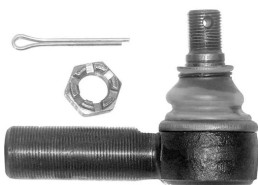
06911VLT наконечник рулевой RHT M30x1,5 / M20x1,5 ISUZU FSR90/FSR34
