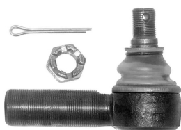
06317VLT наконечник рулевой LHT M30x1,5 / M27x1,5 L=120mm, K=32 [0014607948] [38552 VLT]
