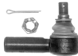
06390VLT наконечник рулевой RHT M30x1,5 / M20x1,5 L=140mm, K=26 [1342026]
