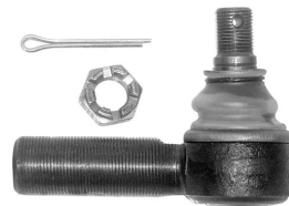
06324VLT наконечник рулевой RHT M30x1,5 / M24x1,5 L=120mm, K=31,5 [1698557] [59134 VLT]
