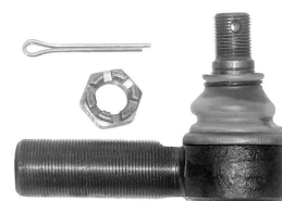
06730VLT наконечник поперечной тяги АМАЗ-206,226 (RHT M30°1,5мм, резьба на пальце M20мм), [SF4863S]
