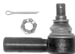
06318VLT наконечник рулевой RHT M30x1,5 / M24x1,5 L=135mm, K=32 [20581089]
