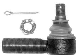
06319VLT наконечник рулевой LHT M30x1,5 / M24x1,5 L=135mm, K=32 [207100008]
