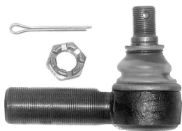
06009VLT наконечник рулевой LHT M30x1,5 / M20x1,5 L=115mm, K=26 [0003300148]
